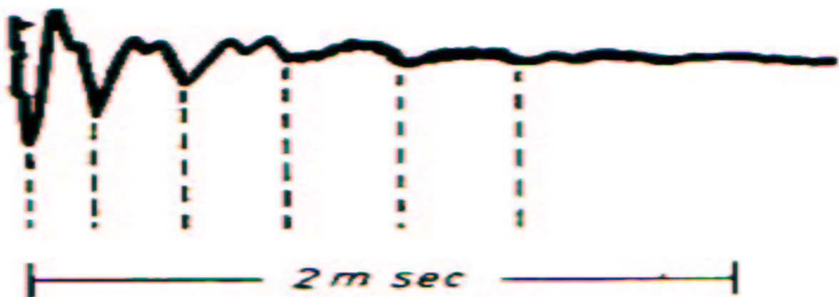
Abb. 4 „Atmospherics“ (Reflexion an Ionosphäre und Erdoberfläche, wie bisher angenommen, oder elektrostatische longitudinale Schwingung?)
